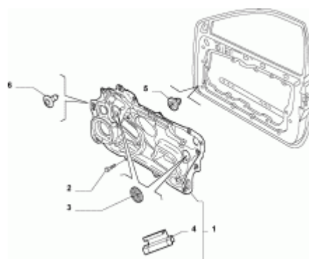
70129/00 - SIDE FRONT DOORS (Var.:2/Rev.:0)
